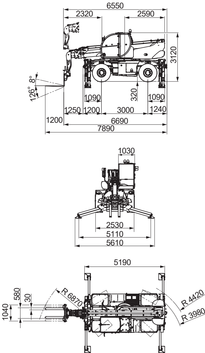
Mit Lastgabel
